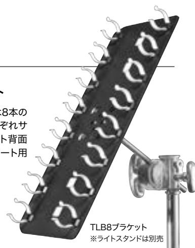
TL60/TL120 用ブラケット
