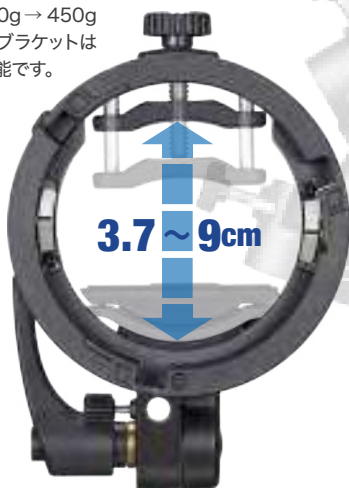
〈新型〉S3 ブラケット 重量：450g
