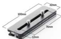
カメラプレート モノボールフィックス 100 (4961360089455) ¥11,000 ■46g ■1/4"J
